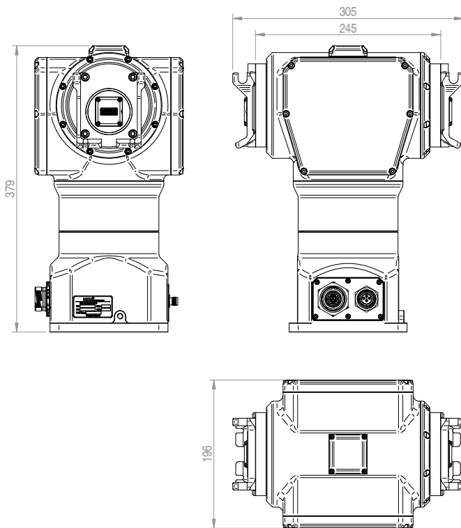
PTU-M dimensions
